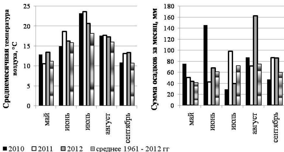
Рис. 1. Метеорологические условия 2010–2012 гг. в Пушкинском филиале ВИР (Ленинградская область)
